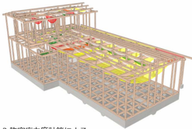
3,許容応力度計算による 中スパン空間の耐震等級判定
